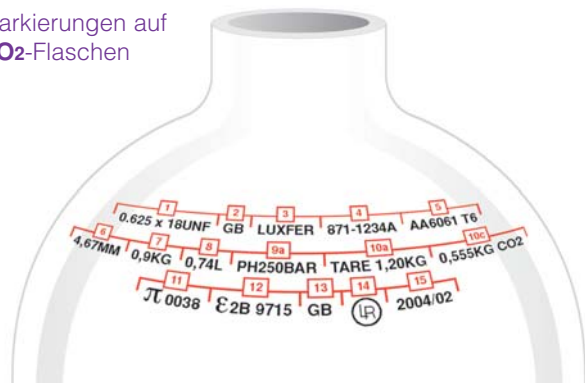
Markierungen auf Druckluft-Flaschen
